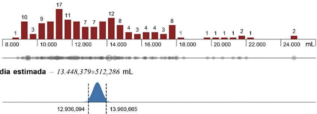
Figura 2. Distribuição do volume (mL) dos membros e médias estimadas.
